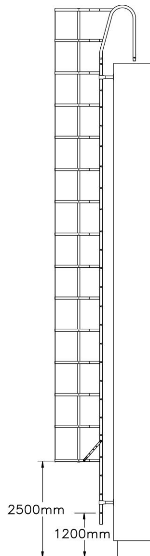
Kuva 2. Selkäkaari mittakuva
