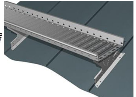
Kuva 3. SK-KAT tai CL-KAT Saumapelti- tai Classic-katto
