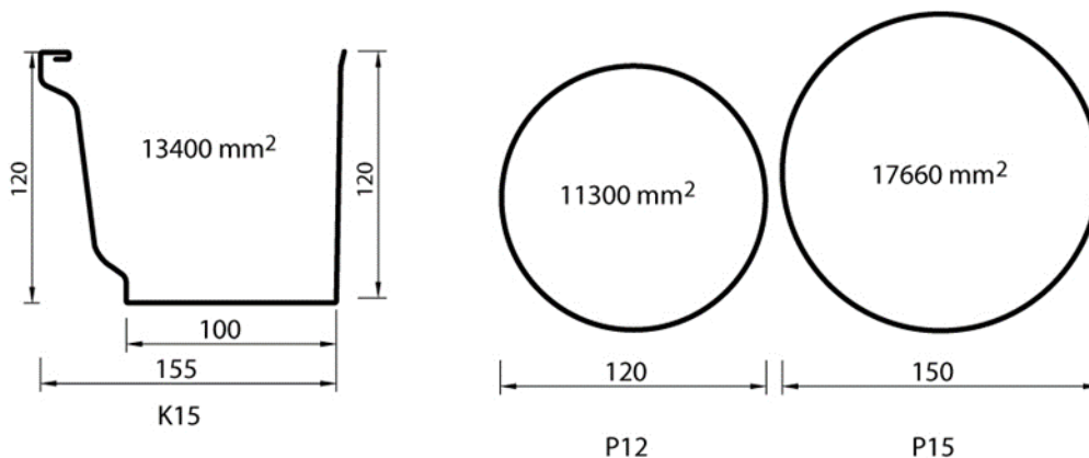
Kuva 1. Läpileikkauspinta-alat
