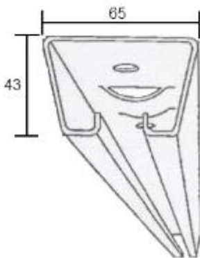
Kuva 1. Nousukisko
