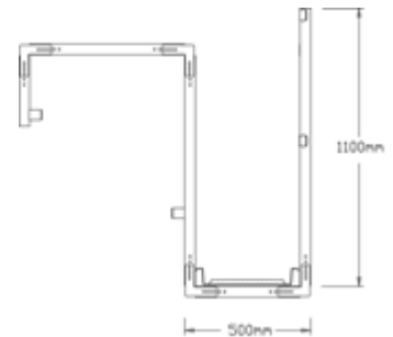
Bild 3. Tvärsnitt av plattformen
