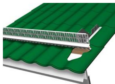
Kuva 2. VARMA 180 tiilikatonle
