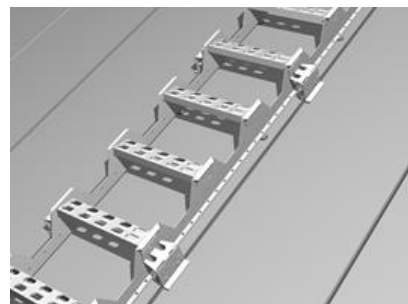
Kuva 3. Kone- ja lukkosauma-katto
