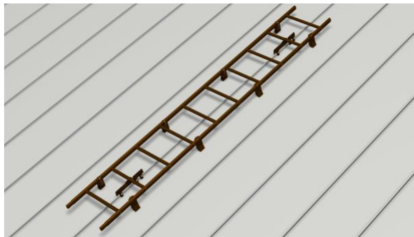
Kuva 4. Lukkosaumakatto
