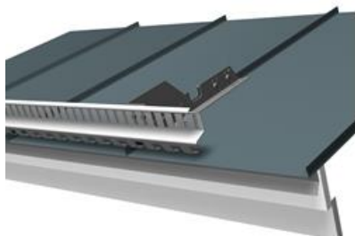
Kuva 1. VARMA 120 konesaumakatolle
