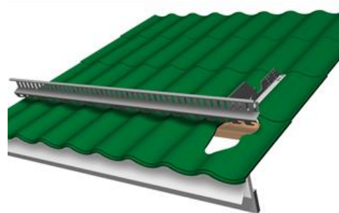
Kuva 4. VARMA 120 muotokatteelle
