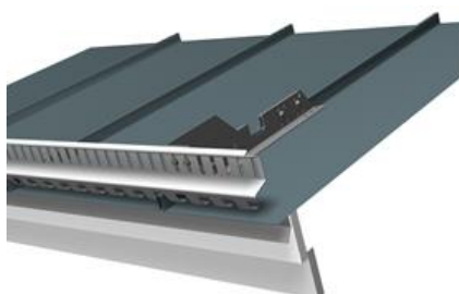
Kuva 1. VARMA 120 konesaumakatolle
