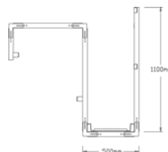
Kuva 3. Leikkauskuva tasosta
